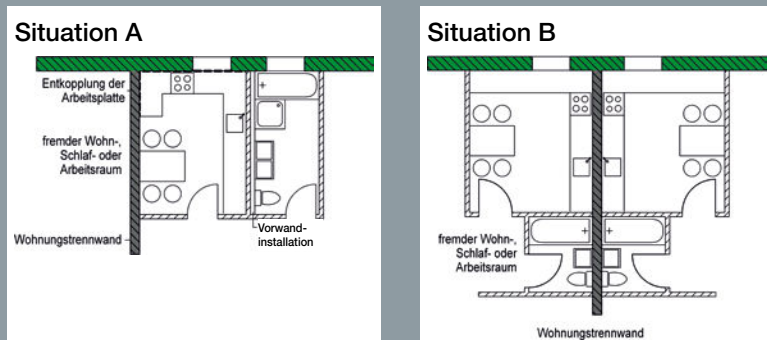
Bild 1.4: Ungünstige Anordnung und Diagonalposition (Bild 1.4 Situation B) lauter Räume an einer Wohnungstrennwand [5].
