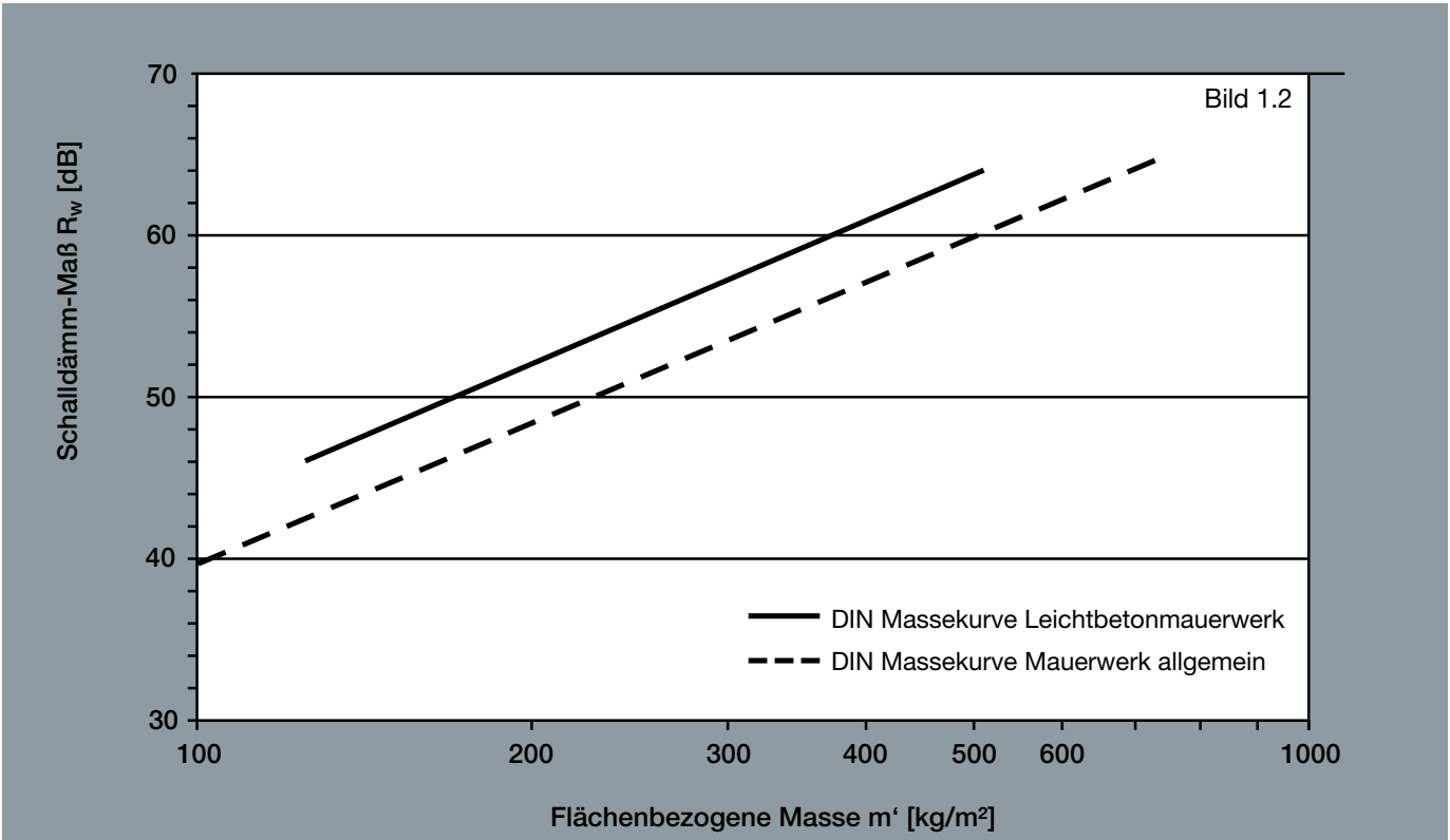
Bild 1.2: Schalldämmung von Leichtbetonmauerwerk in Abhängigkeit der flächenbezogenen Masse. Im Bereich von m' 140–480 kg/m 2 ist das Schalldämm-Maß R_w um 2 dB höher als von Mauerwerk allgemein.
